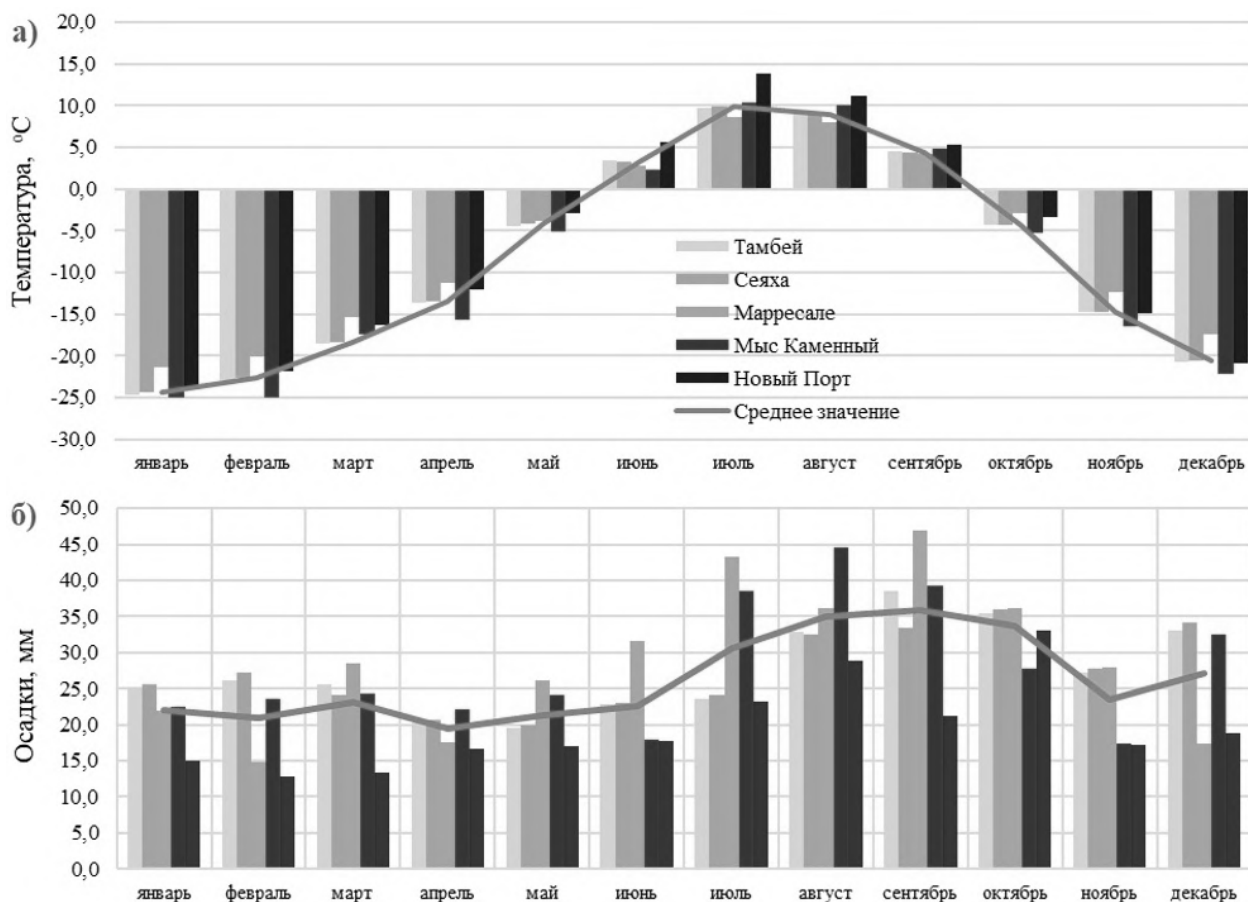
График годового хода температур (а) и осадков (б) за период 1985–2023 гг. по данным метеостанций на территории полуострова Ямал.
