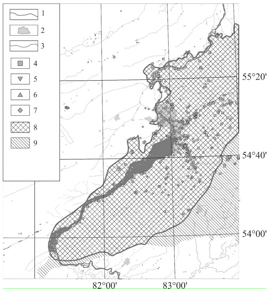
Распределение величин радиевого эквивалента ( Ra_{eg} ) в природных водах изучаемого региона. Фрагмент Государственной геологической карты и схематический разрез Обь-Зайсанской складчатой области (с упрощением) [Бабин и др., 2015].
