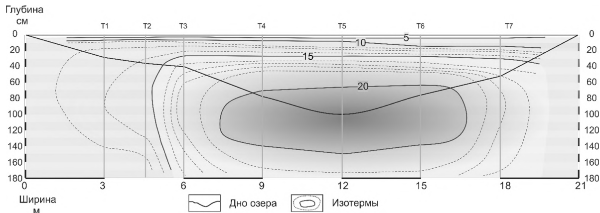
Распределение температуры в толще воды и донных отложениях оз. Мохсоголлох 20.09.2025 г.
