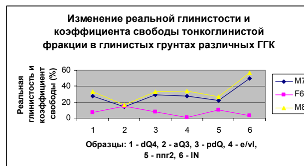
Рис. 2. Изменение параметров микроструктуры в глинистых грунтах.
