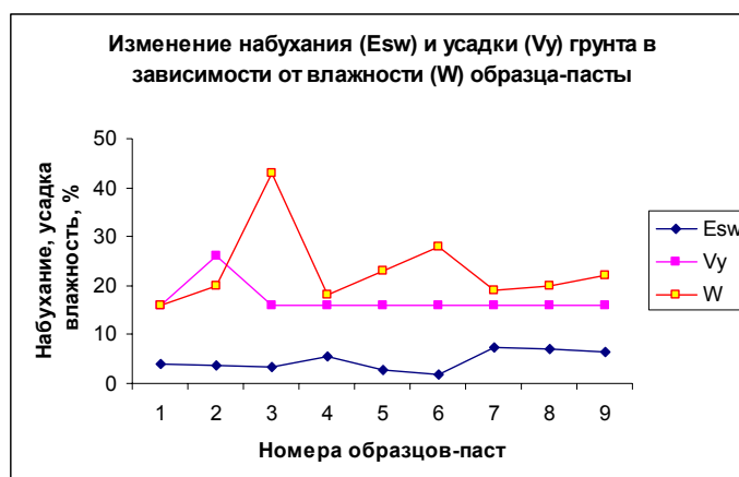
Рис. 6. Изменение набухания и усадки грунта (лабораторный эксперимент).
