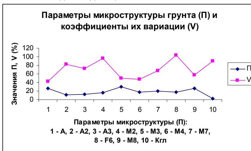
Рис. 3. Характер распределения параметров микроструктуры в глинистых и лессовых грунтах по данным общей выборки (n=91).
